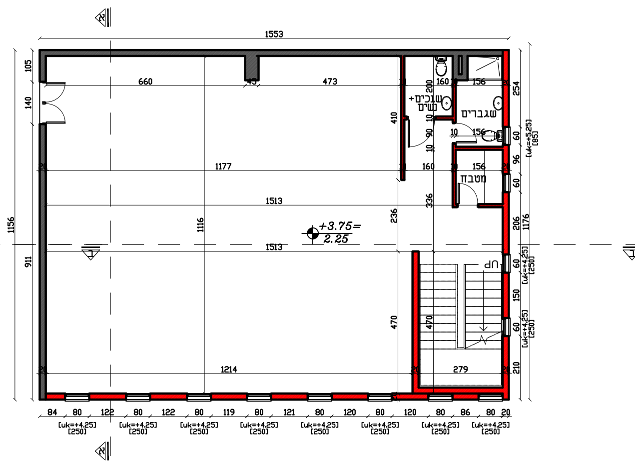
תכנית קומת א קנ"מ 1:100
