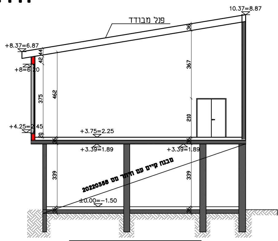
חתך א-א קנ"מ 1:100
