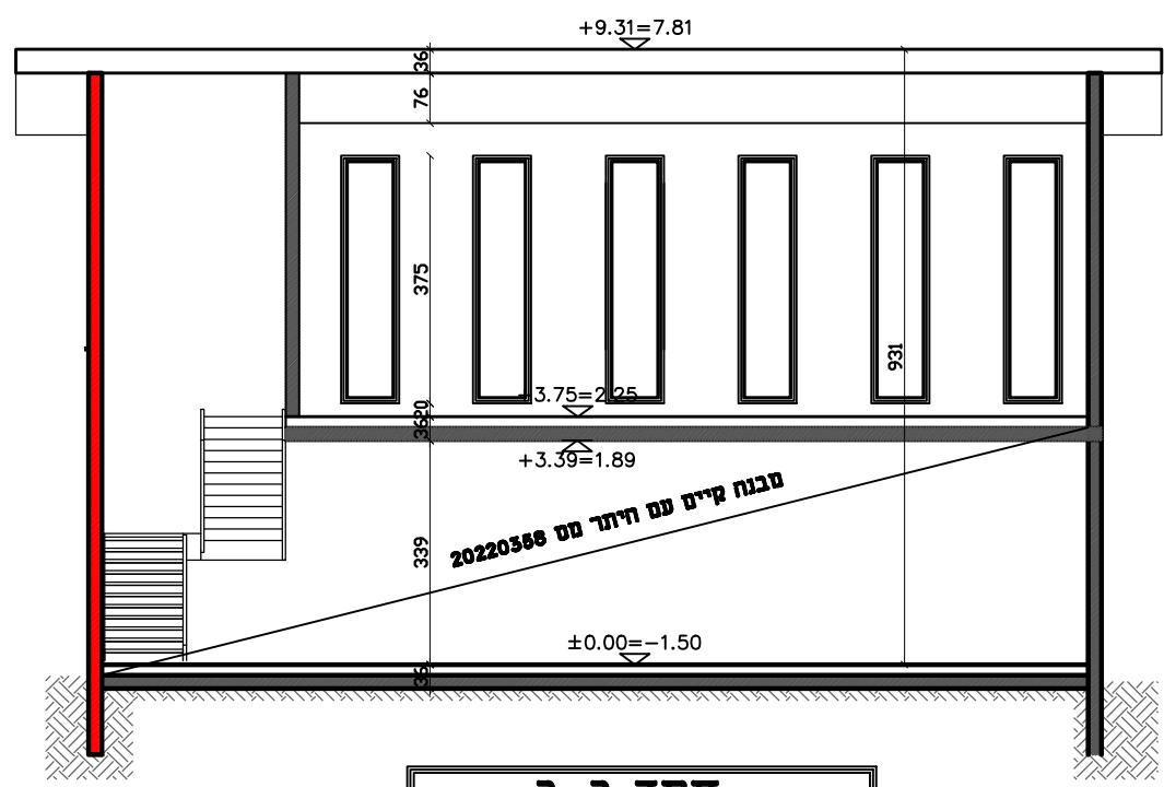
חתך ב-ב קנ"מ 1:100
